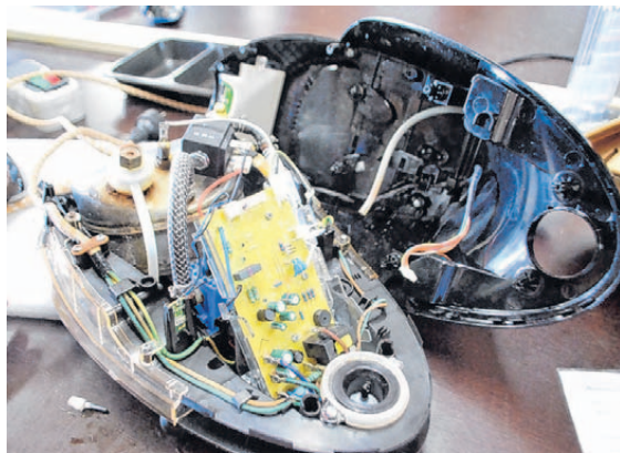
Im Innern des Dampfbügeleisens sind braun verfärbte Stellen zu sehen. Sie zeigen an, dass es in dem Elektrogerät eine undichte Stelle gibt, wo Wasser austritt.
